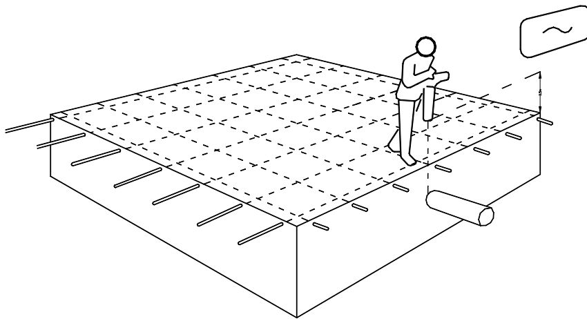
图 e 钢筋网下管道探测示意图
