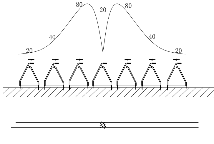
A 字架读数示意图
