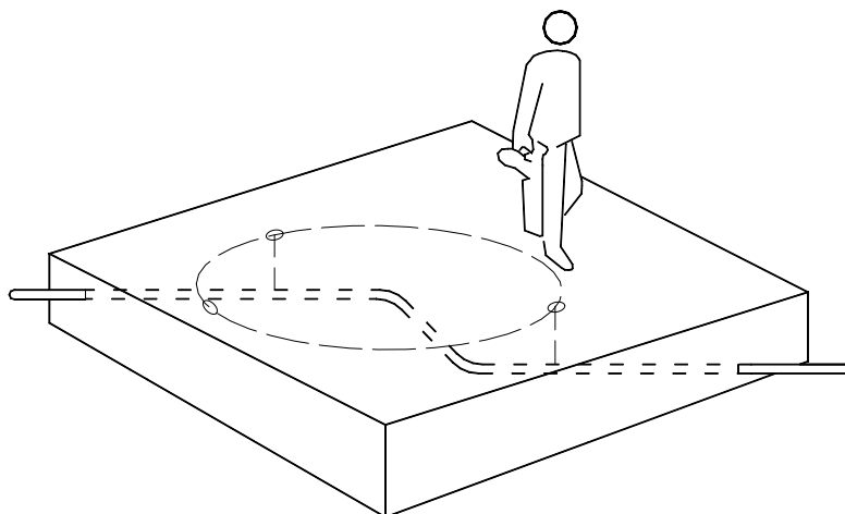
图 a 管道变深探测示意图
