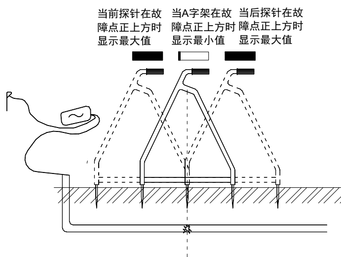
A 字架对管线故障点定位示意图
