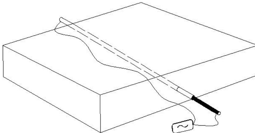
图二十六 双端连接法示意图
