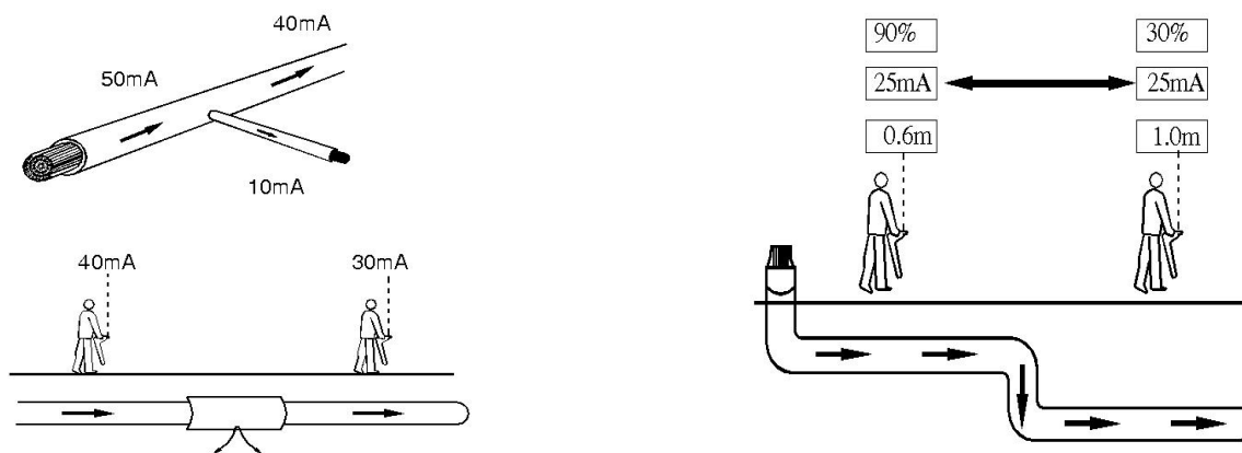
图 g 三通和弯头处电流测量示意图
