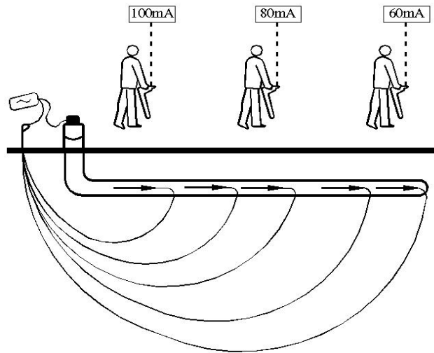
图 h 电流测量原理示意图
